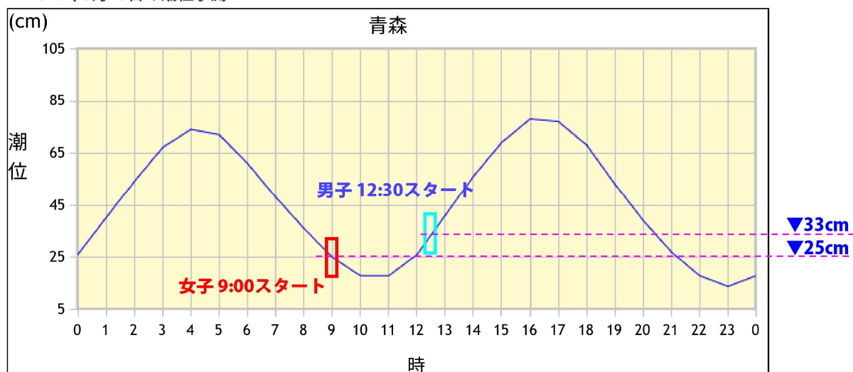
毎時潮位グラフ 青森 2026年9月13日の潮位予測
